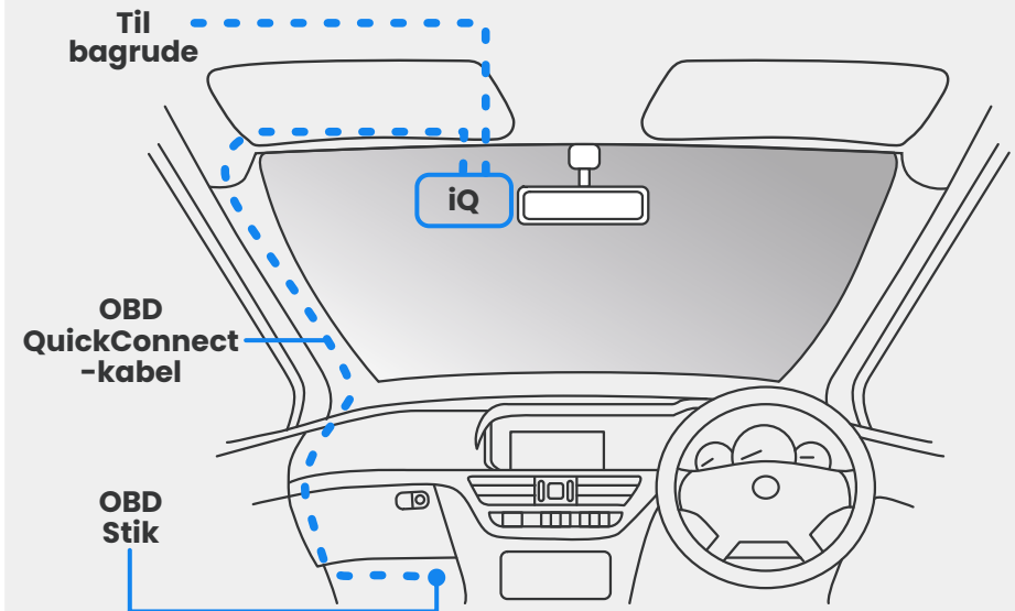
Omtrentlig placering af iQ-, OBD- og QuickConnect-kabel.
